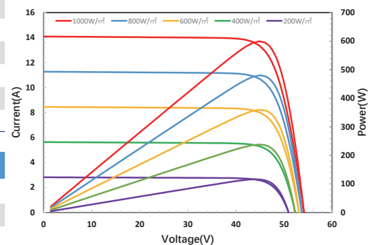
电流-电压曲线及功率-电压曲线 (600W)
